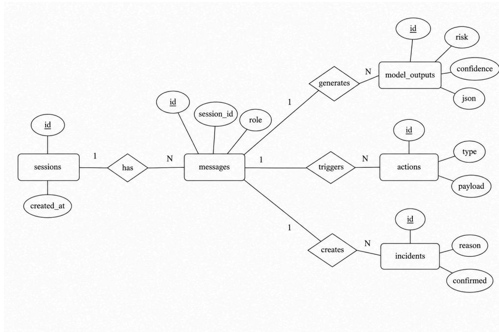
Figure 3.2: ER diagram
